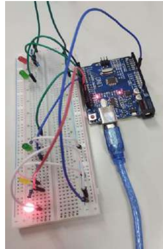
Grupo de estudiantes reconociendo los componentes del kits de robótica. Placa Arduino con proyecto desarrollado por los estudiantes
